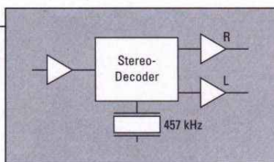
Absolute Stereo-Kanaltrennung durch Keramik-Resonatoren im PLL-Stereodecoder.
