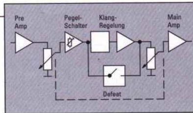
Rauschminimierung durch doppelte Lautstärkeregelung.
