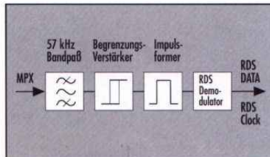
RDS-Modul.
