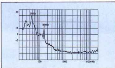
Wiedergabe-Fremdspannung mit herkömmlichem Trafo.
