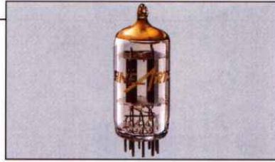
Hochwertige Spanngitterröhren E 83 CC.
