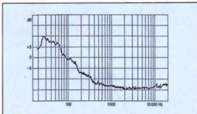
Wiedergabe-Fremdspannung mit Schnittbandkern.
