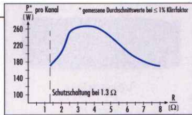
Ausgangsleistung A-9009.
